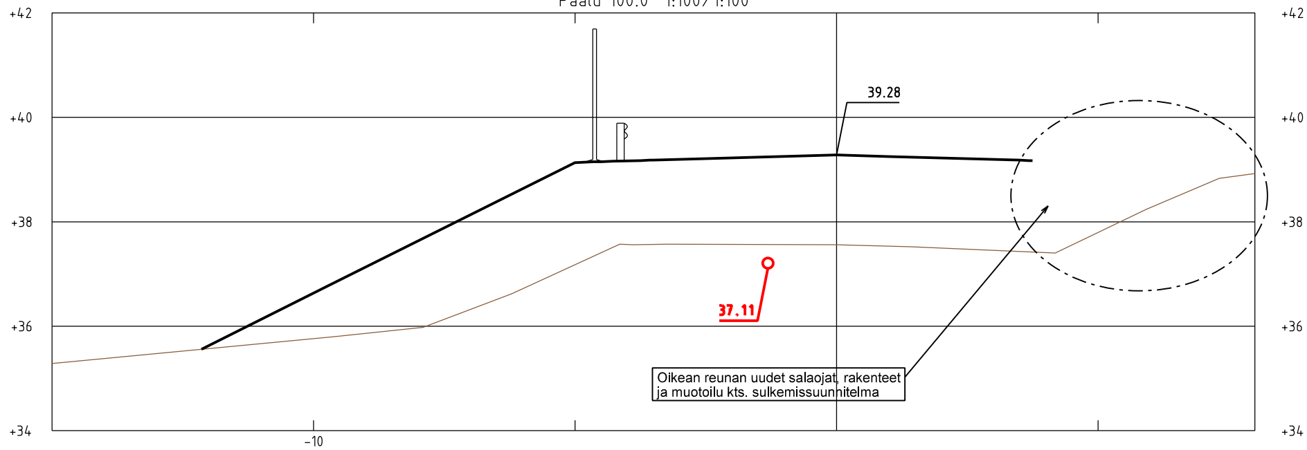
Paalu 100.0 1:100/1:100
