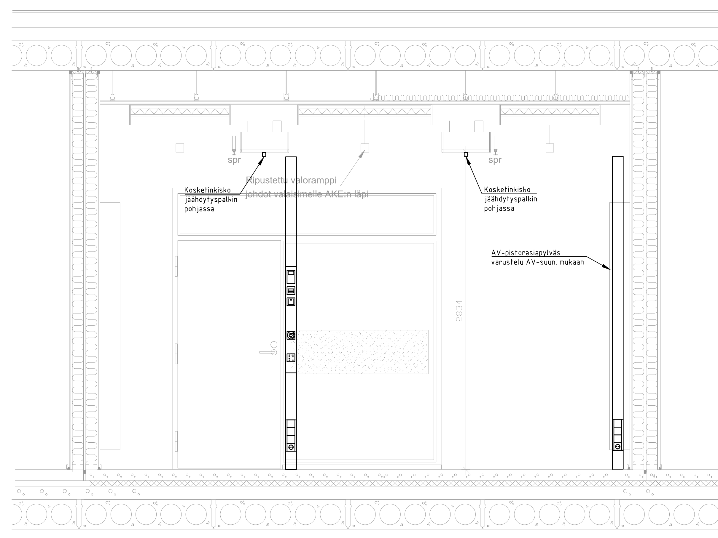
leikkaus B-B
