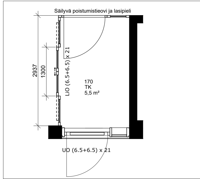
Pohjapiirros 170 Tuulikaappi
