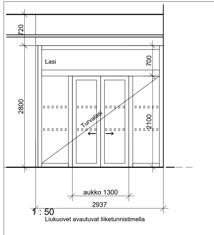
Tuulikaapin liukulasiseinäkaavio
