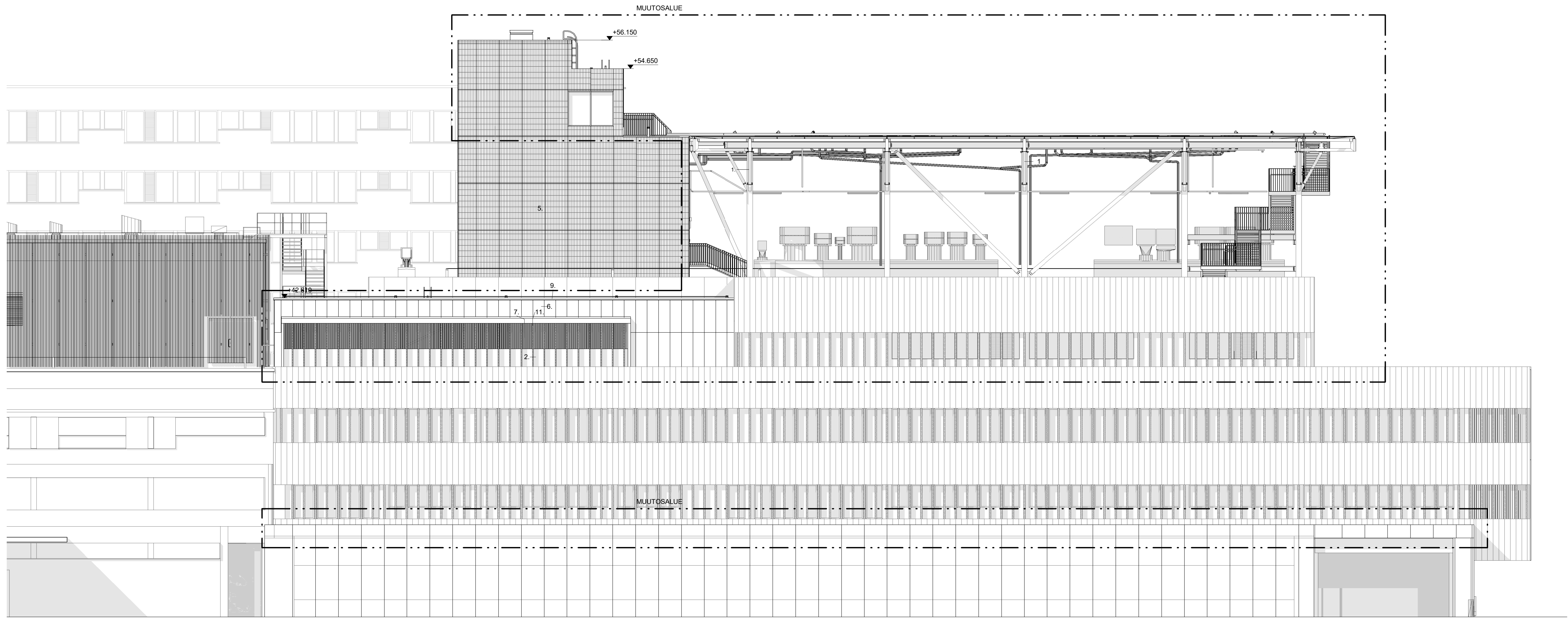
Julkisivu, Itään 1 : 100
