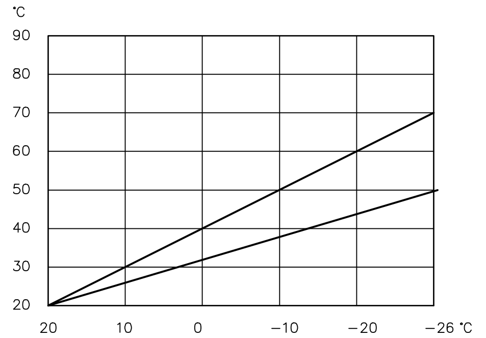
TV1 PATERILÄMMITYS TOIMINTALÄMPÖTILAT
