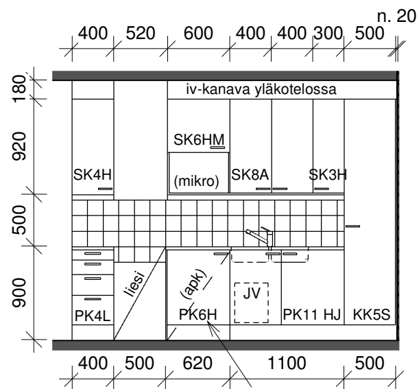
SEINÄ 2 1 : 50
