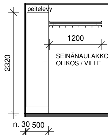
EDESTÄ 1 : 50
